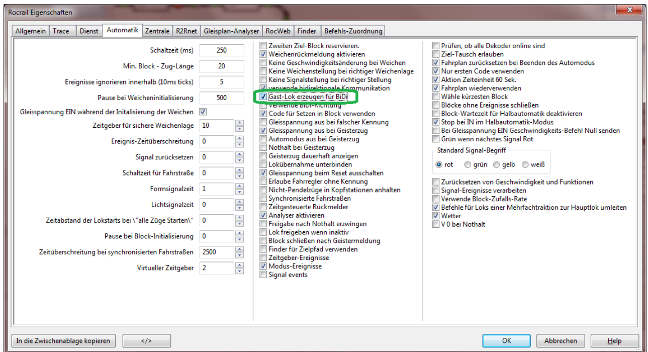
Abbildung 14 Rocrail – Gast-Lok
