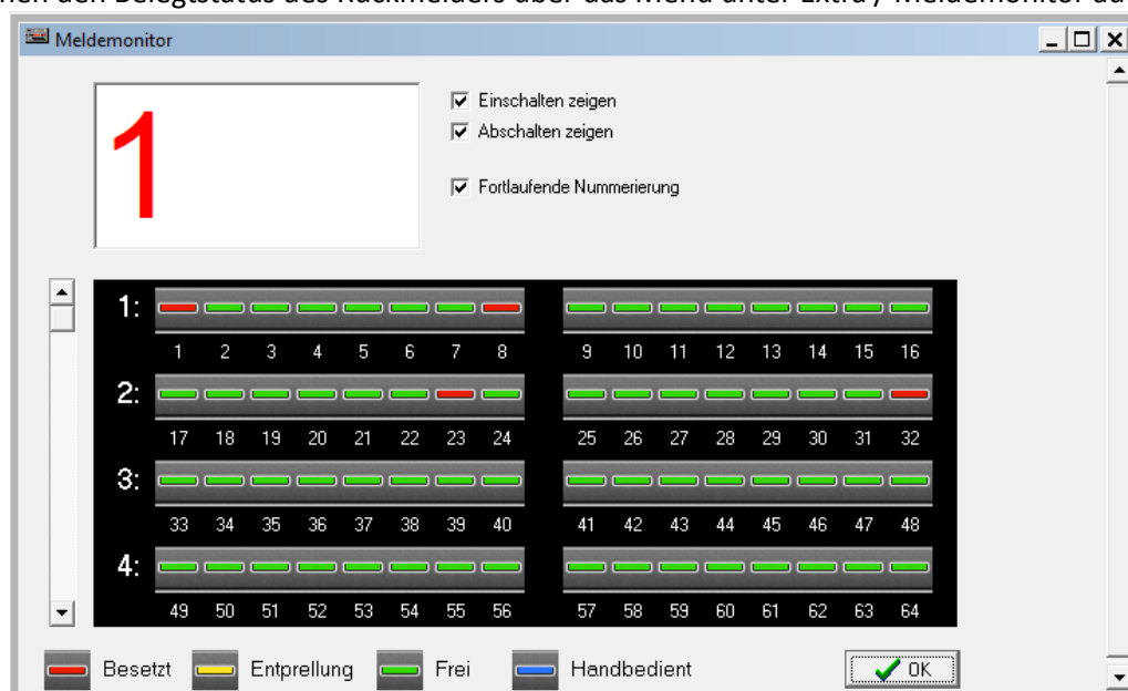
Abbildung 27 ModellStw - Meldemonitor
