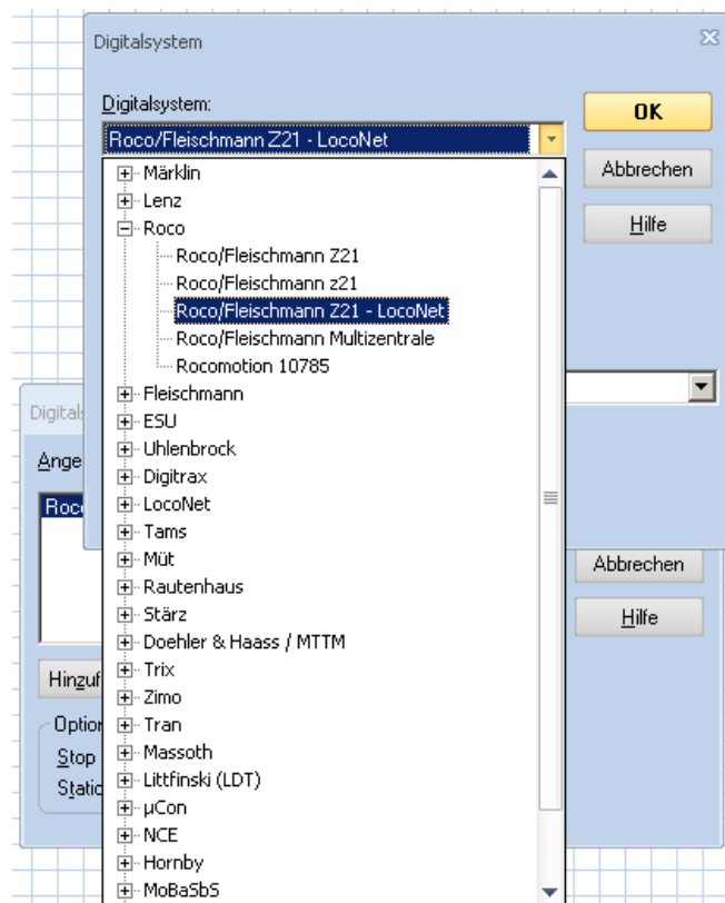
Abbildung 18 TrainController - Z21-LocoNet-Bus
