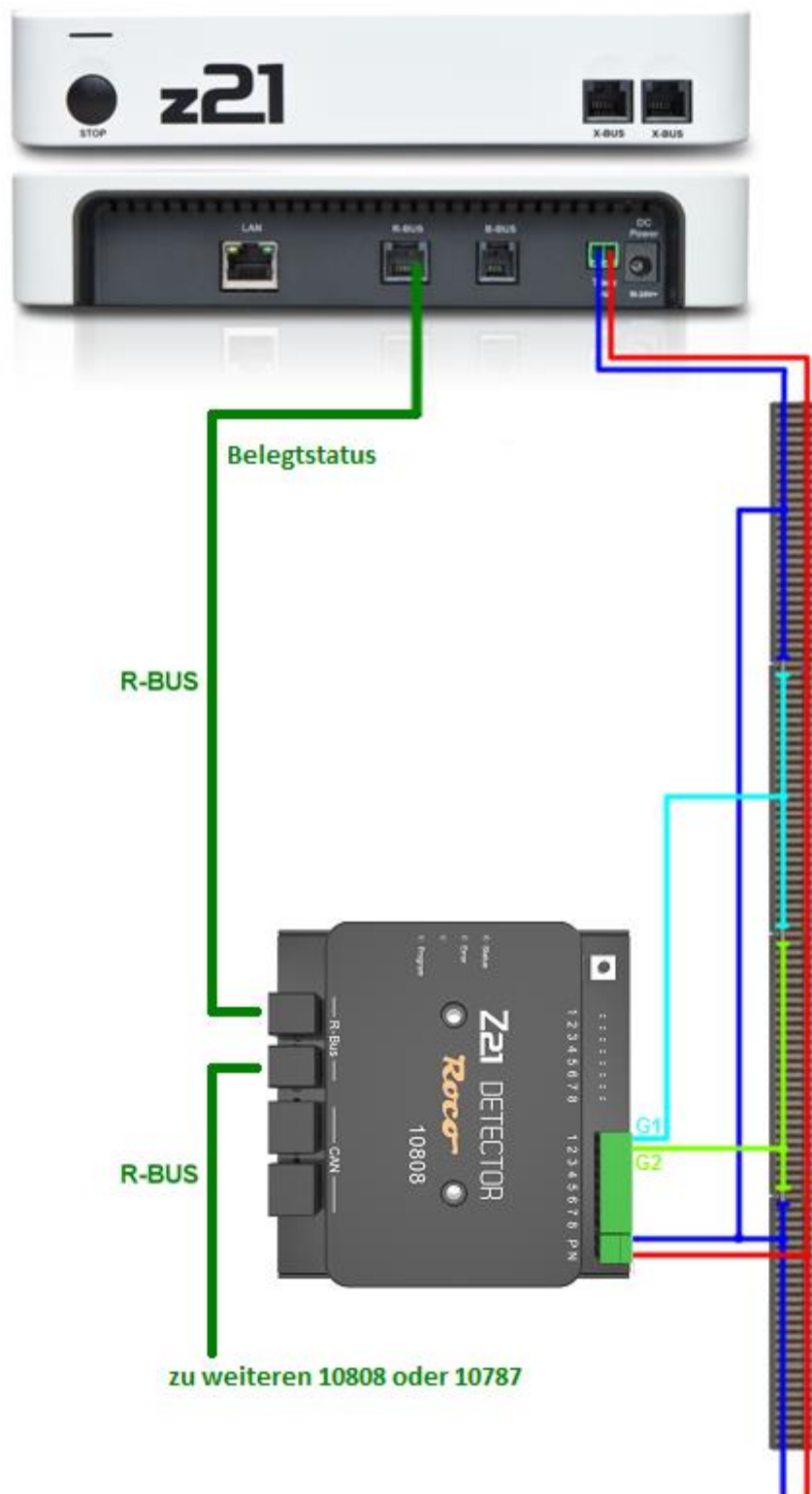
Abbildung 3 10808 über R-BUS an z21 und z21start
