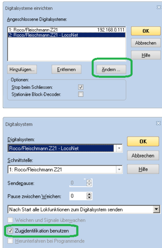
Abbildung 19 TrainController - Zugidentifikation aktivieren
